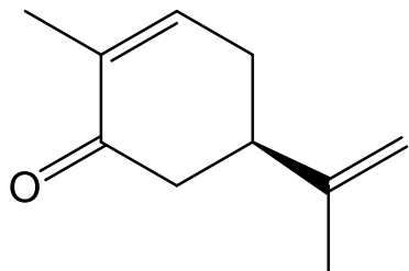
R-carvone
