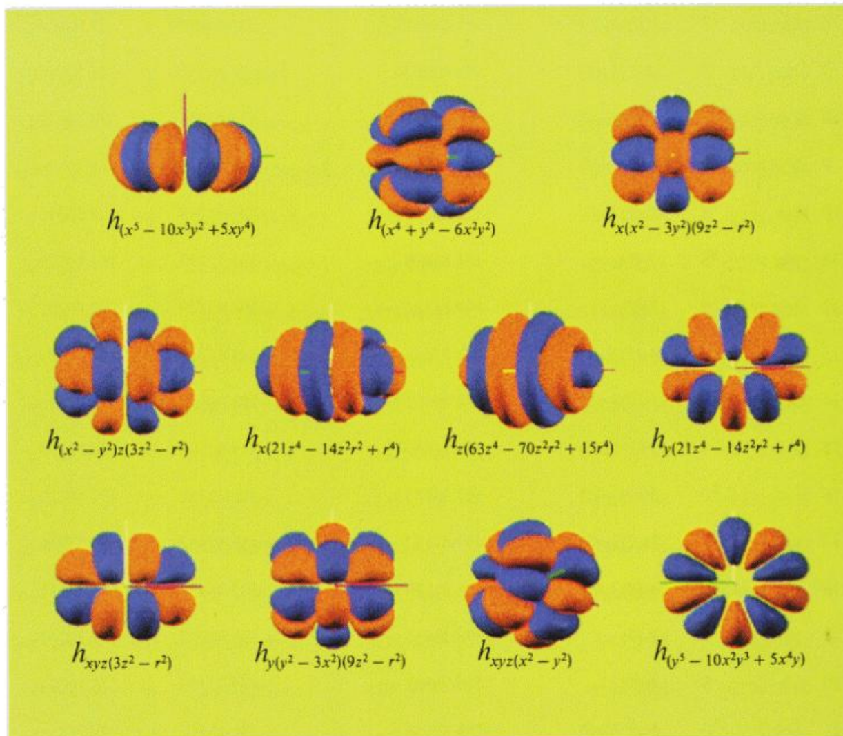
Representação 3D-dimensional dos orbitais do tipo h.
